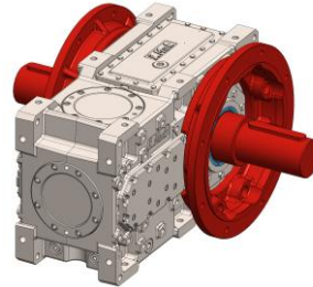
MA / MK .... FD-SD Double output flange-Double output solid shaft Bride de sortie double - Arbre de sortie double
